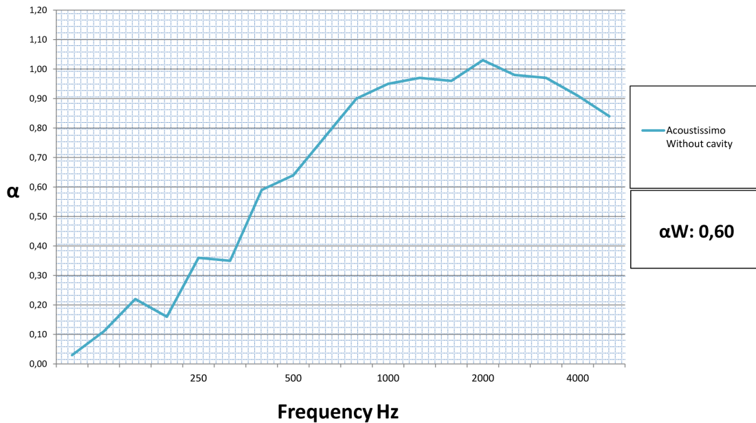
Acoustissimo Without Cavity NF EN ISO 11654
