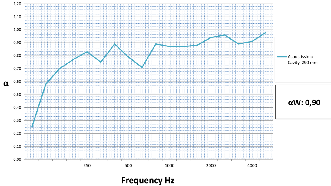
Acoustissimo 290 mm - Cavity NF EN ISO 11654
